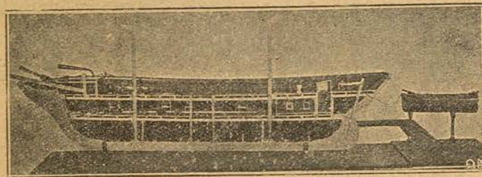
Τομῆ πυρπολικῶ.
