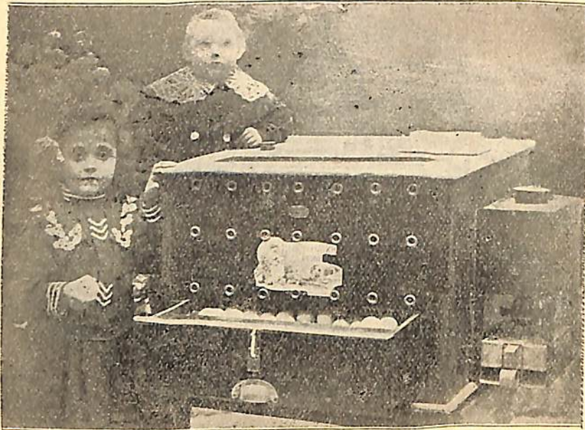
Εἰκ. 32. Κλωσσομηχανὴ διὰ θερμοῦ ὕδατος.
